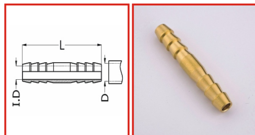
雙頭插心 Union
